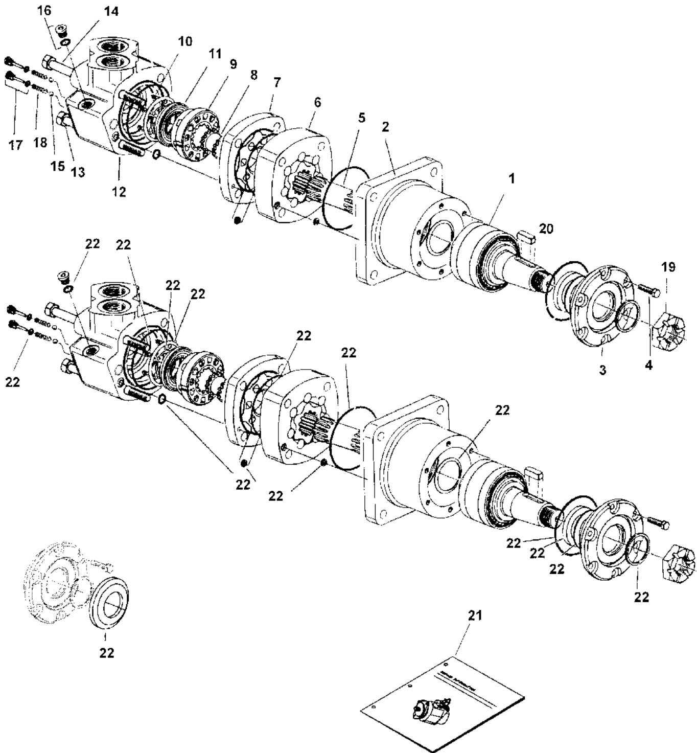
FIG. 1 - MOTOR BREAKDOWN (PART # 22626)
